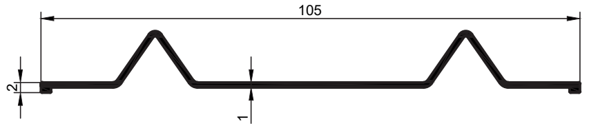
16024 0,394 Kg/Mt
