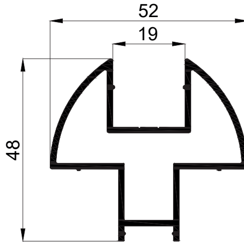
16756 0,859 Kg/Mt
