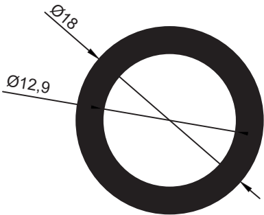
16457 0,345 Kg/Mt
