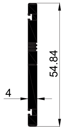
16724 0,577 Kg/Mt
