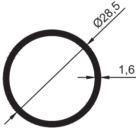
16456 0,380 Kg/Mt
