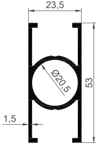
16142 0,739 Kg/Mt
