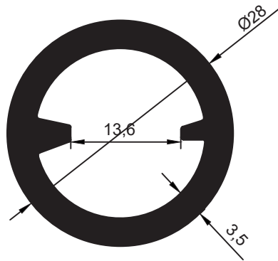
16459 0,795 Kg/Mt
