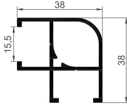
16145 0,650 Kg/Mt
