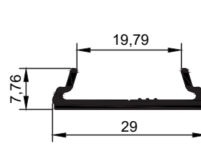
16732 0,193 Kg/Mt
