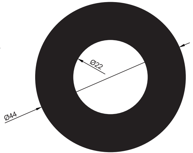
16458 3,095 Kg/Mt
