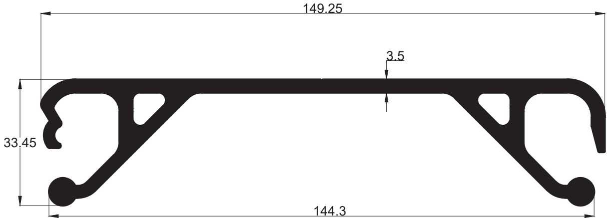
16954 2,832 Kg/Mt
