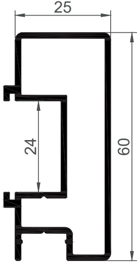
16146 0,830 Kg/Mt
