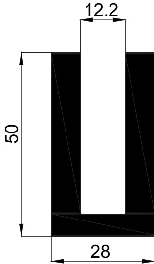
16616 0,591 Kg/Mt
