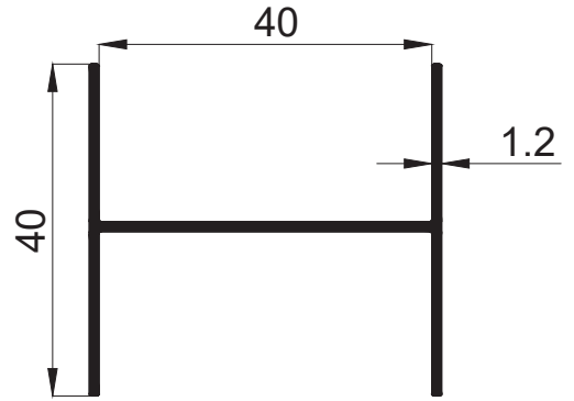
16356 0,395 Kg/Mt
