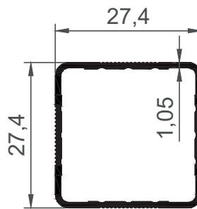
16128 0,294 Kg/Mt
