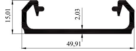
16715 0,514 Kg/Mt
