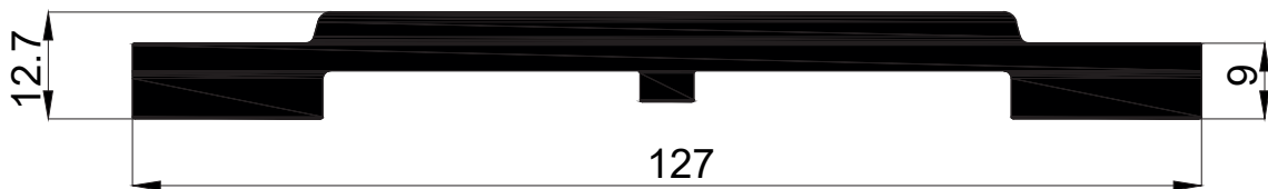
16736 2,730 Kg/Mt
