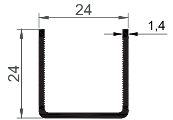
16306 0,244 Kg/Mt
