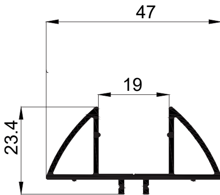
16754 0,455 Kg/Mt
