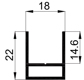
16757 0,248 Kg/Mt
