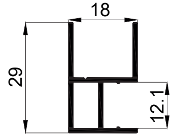
16758 0,294 Kg/Mt
