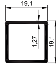
16733 0,247 Kg/Mt
